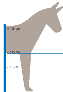
Elektrozaun für Springpferde Empfehlung: Seil, Breitband bis 40 mm
