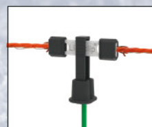
einfaches und schnelles Reparieren durch unsere Litzclip® Reparatursets
