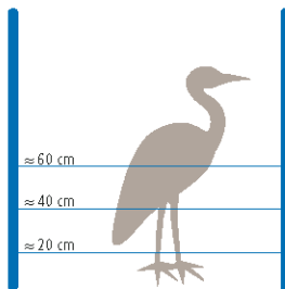
Elektrozaun zur Abwehr von Fischreiher Empfehlung: Hobbyset, Litze
